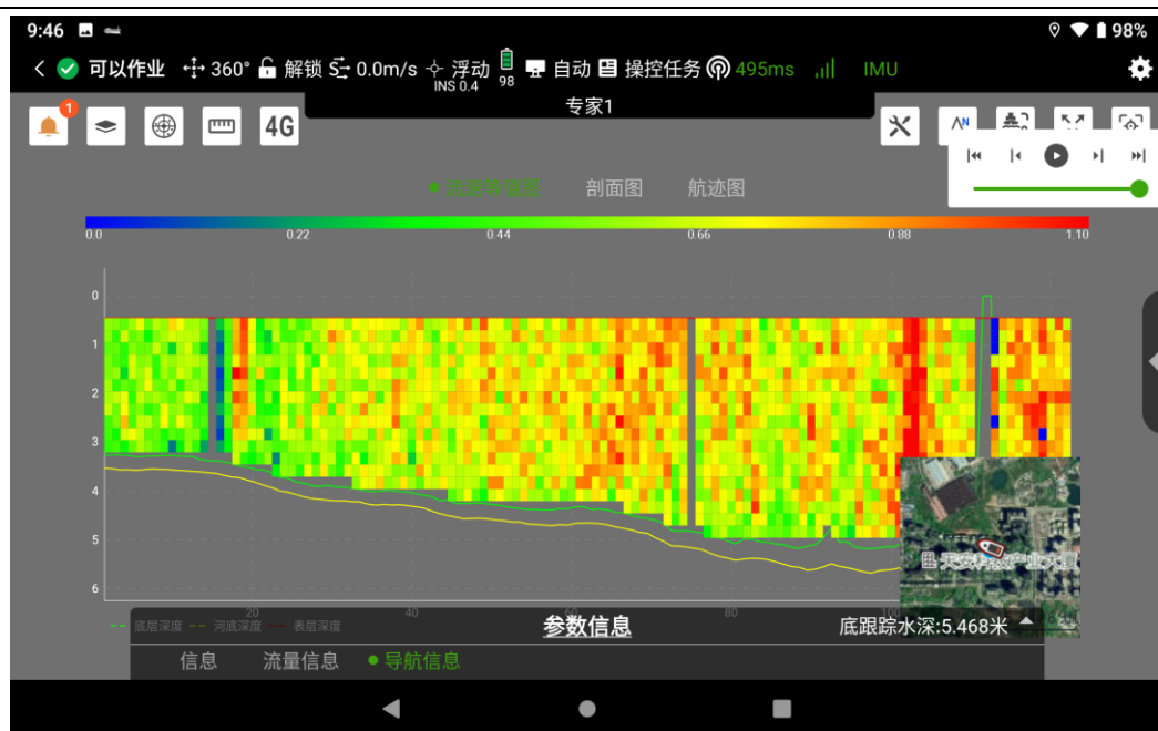
等值流速图
